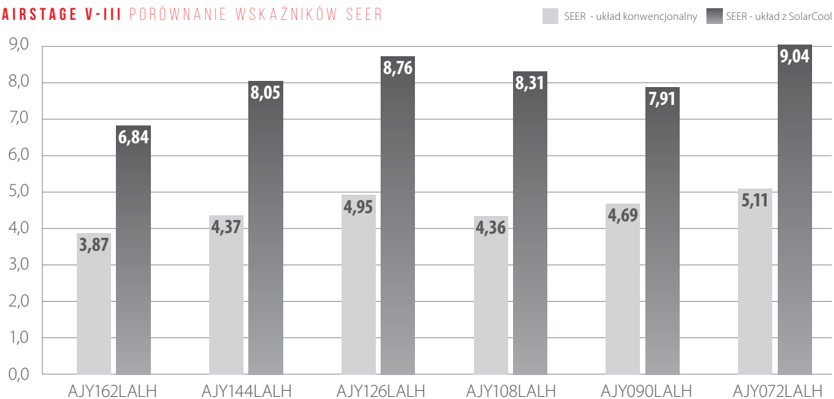
AIRSTAGE V-III PORÓWNANIE WSKAŹNIKÓW SEER
